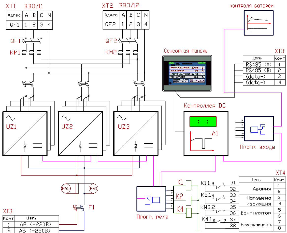
Рис. Однолинейная схема ВЗУ-1
